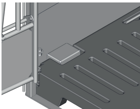
Détail fixations caillebotis
