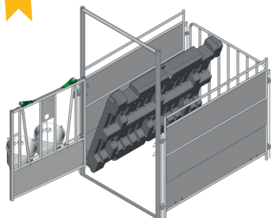
Paroi métallique avec fixations caillebotis
